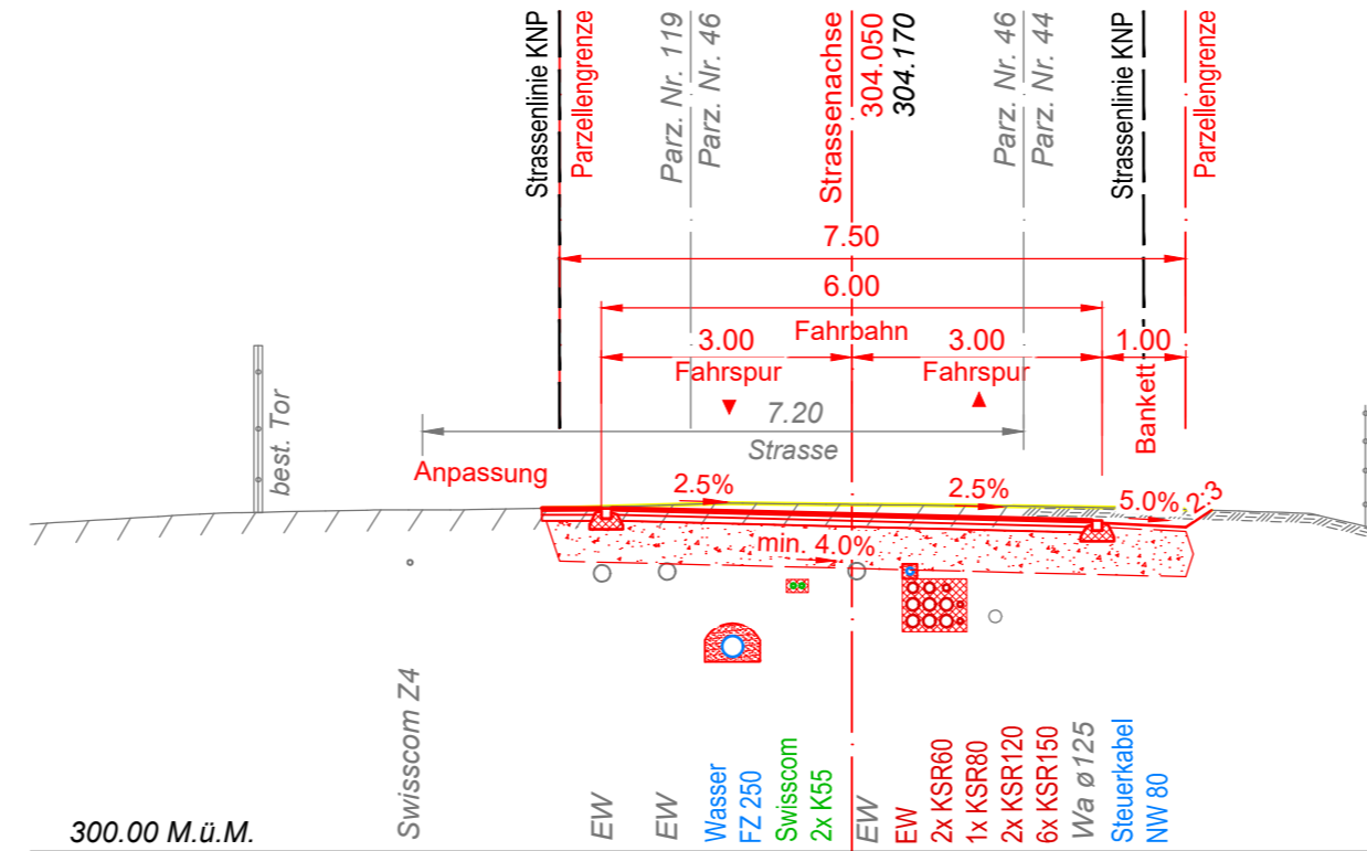
Querprofil 34 1586.00m
