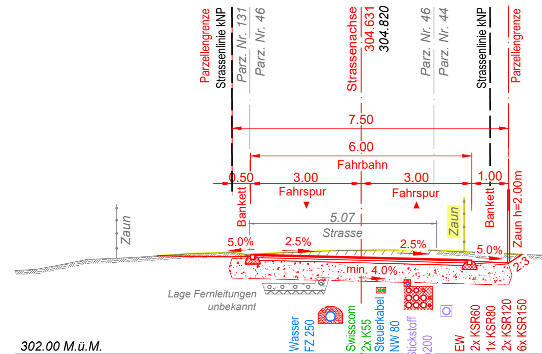
Querprofil 29 1356.00m
