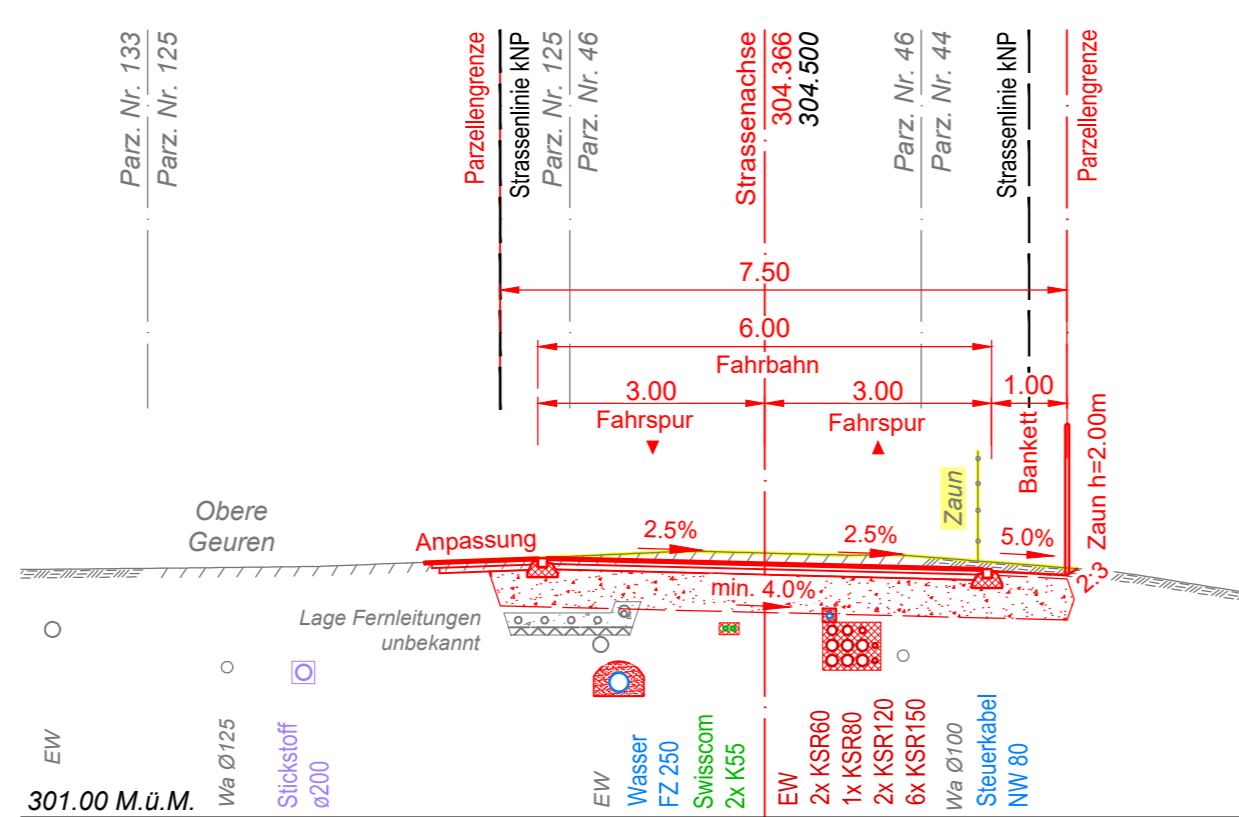
Querprofil 32 1506.00m
