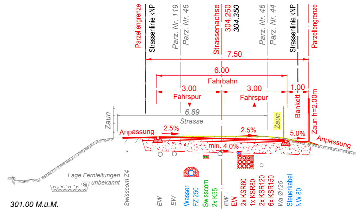
Querprofil 33 1536.00m
