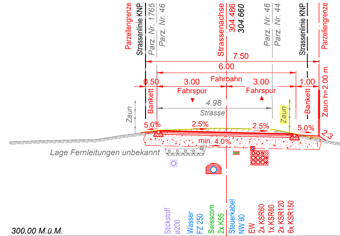
Querprofil 30 1406.00m
