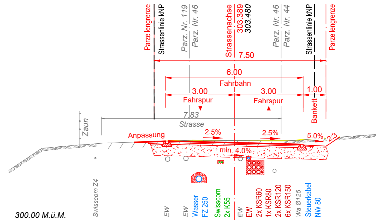
Querprofil 35 1626.00m
