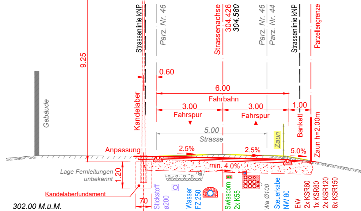
Querprofil 31 1456.00m
